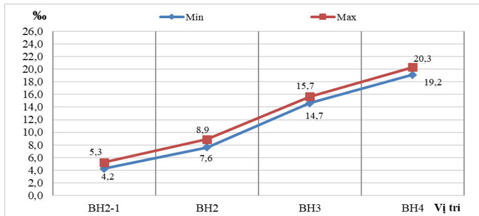
Hình 3: Biểu đồ độ mặn trên sông Bến Hải
