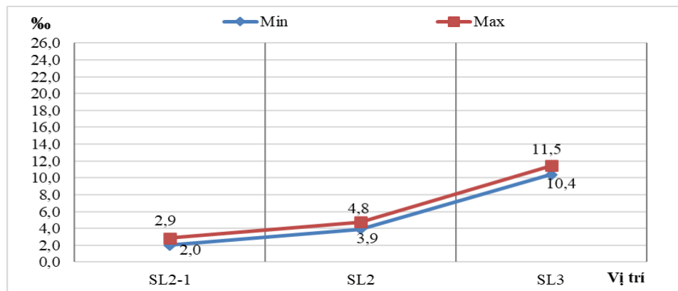
Hình 4: Biểu đồ độ mặn trên sông Sa Lung (Có phụ lục kết quả quan trắc kèm theo)
