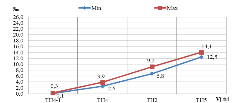
Hình 1: Biểu đồ độ mặn trên sông Thạch Hãn
